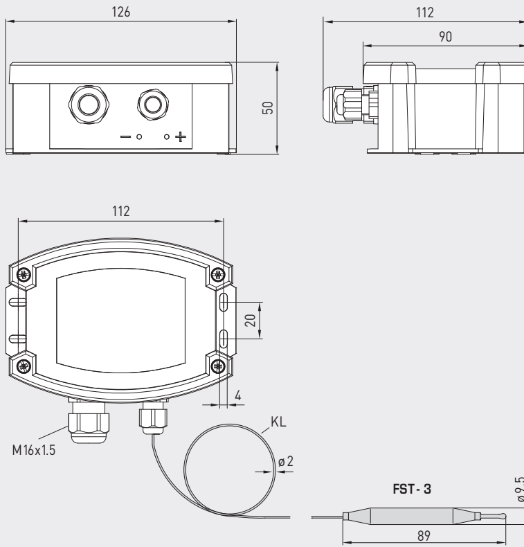
Disegno quotato
