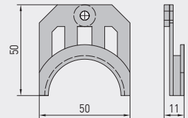
Disegno quotato
