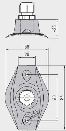
Disegno quotato
